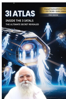
3i Atlas
